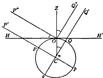
FIG 8 Altitude of the Pole Equals the Observer's Latitude
