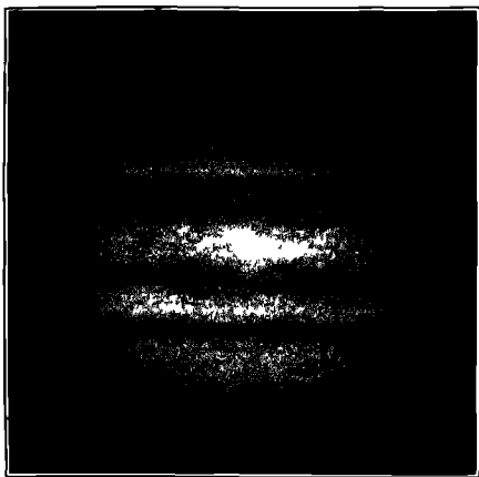
FIG. 149 Jupiter
