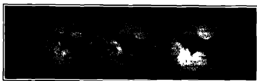
FIG 139 Mars
