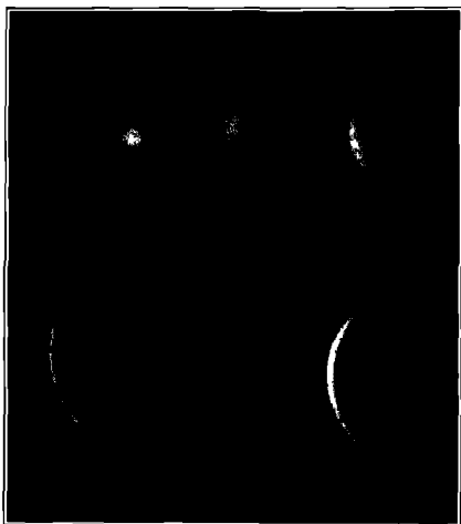
FIG 136 Venus
