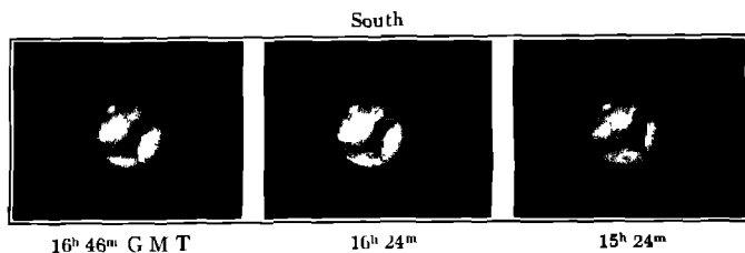
FIG 140 Mars
