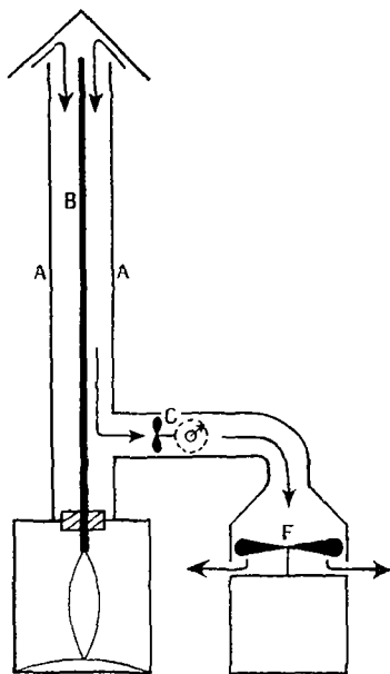
FIG. 1.—Ebert ion-counter.
