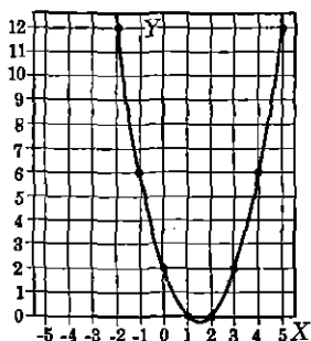
FIG. 16. Graph of y = x^2 - 3x + 2
