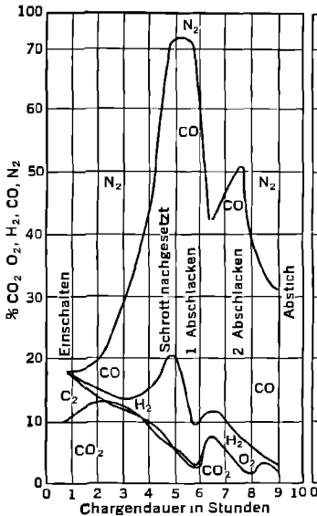
Abb 165 c) Lichtbogenofen
