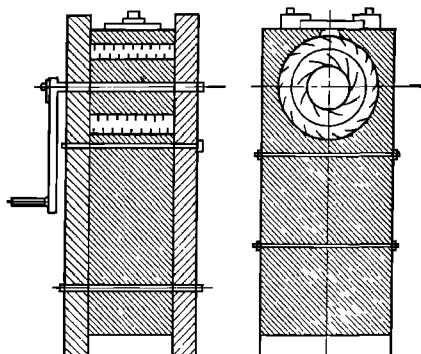
Abb. 162 Pickle (Mastikator) von HANCOCK
