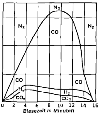
Abb 165 b) Thomasverfahren
