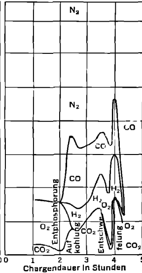
Abb 165 d) Induktionsofen
