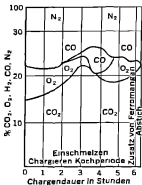
Abb 165 a) S-Martinverfahren
